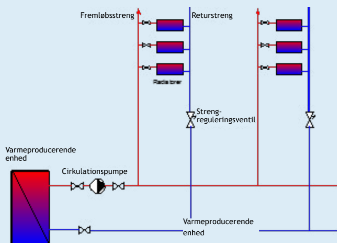
To-strengsanlæg
