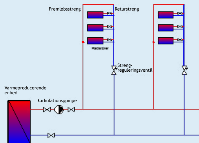
En-strengsanlæg
