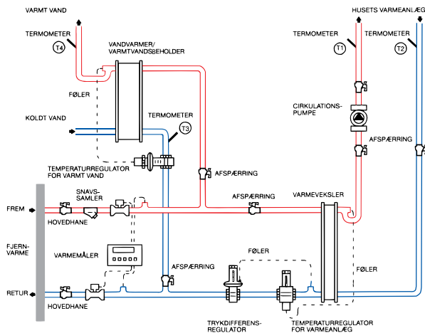
Indirekte anlæg
