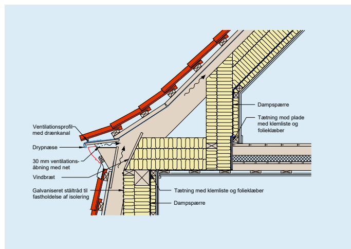
Figur 3: Snittegning i toppen af mansardtaget, hvor det fortsætter i skråtag med skunk.
