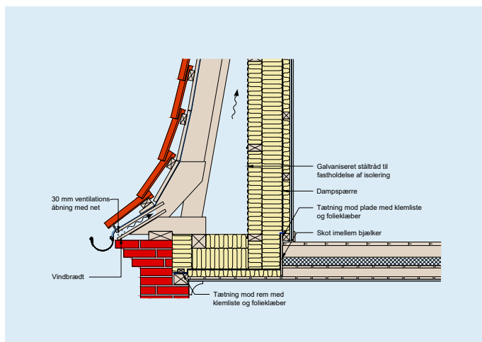
Figur 2: Snittegning i bunden af mansardtaget.
