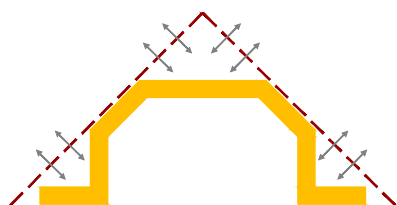
1 ventilationsstuds skiftevis i top og bund af skunkrum og loftsrum
