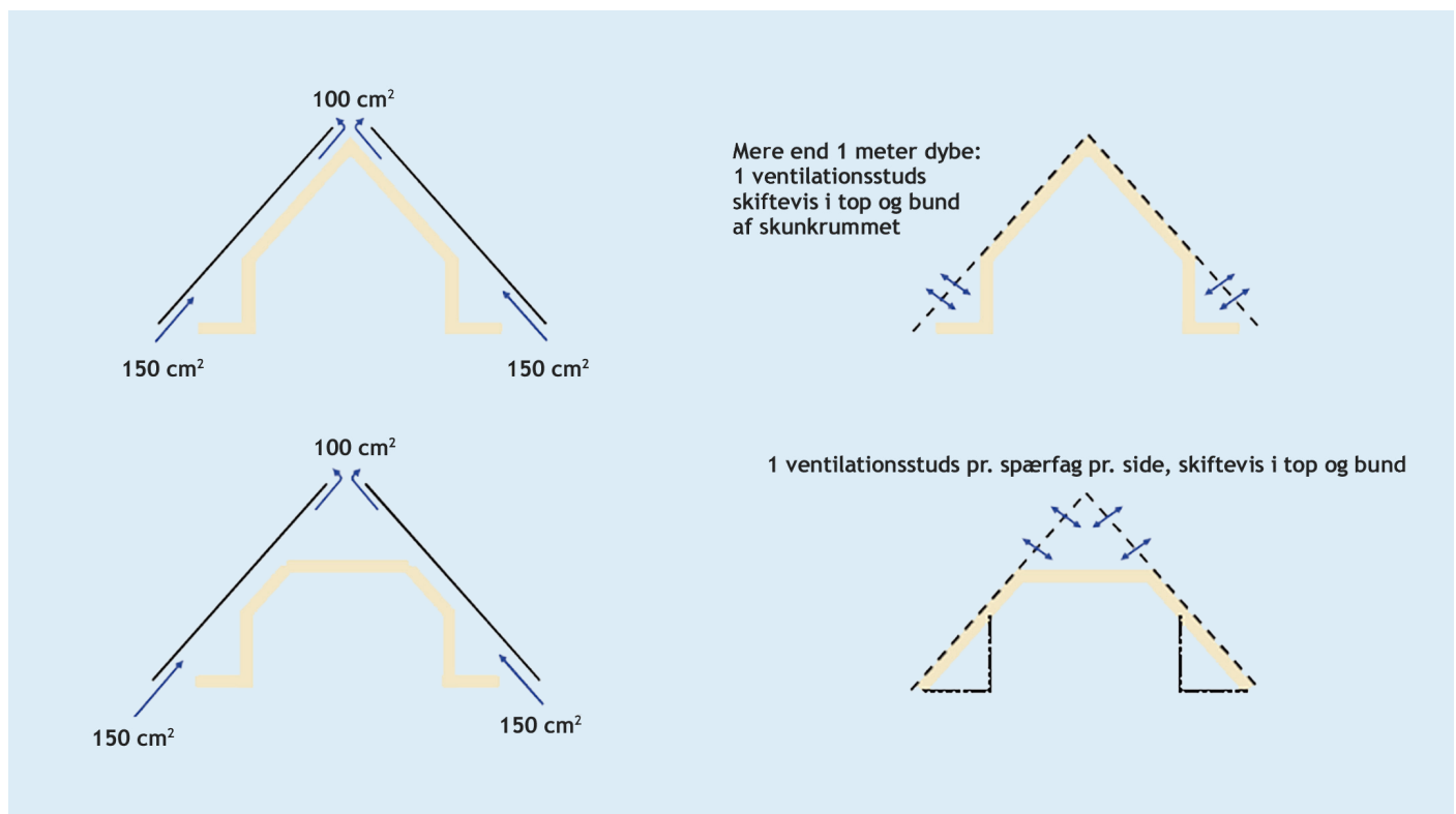
Ventilation af skrå tagflader set i sammenhæng med ventilation af hele tagkonstruktionen - ved diffusionstæt undertag (til venstre) og diffusionsåbent undertag (til højre).
