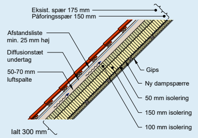
Skråvæg med diffusionstæt undertag og indvendig påføring af spær
