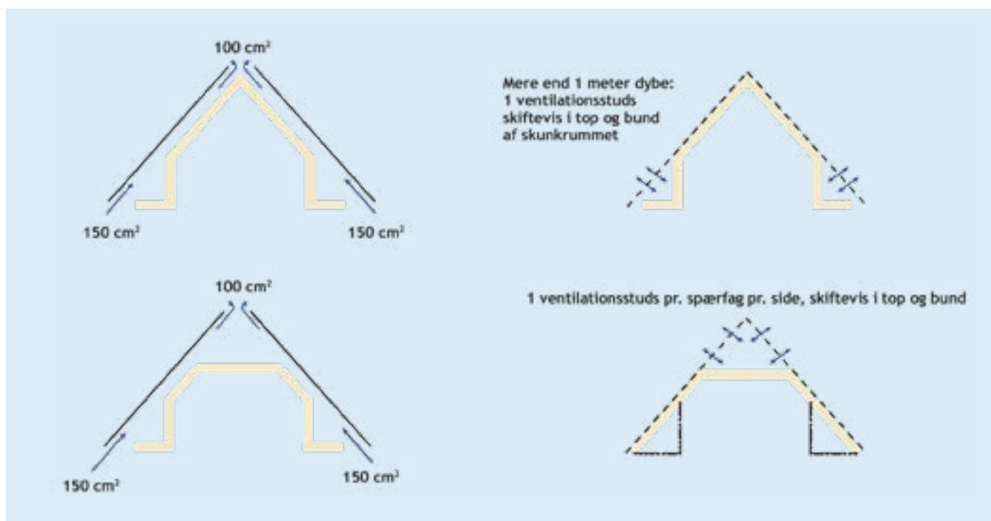
Ventilation af skrå tagflader set i sammenhæng med ventilation af hele tagkonstruktionen - ved diffusionsstæt undertag (til venstre) og diffusionsåbent undertag (til højre).
