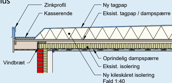
Fig. 1 Koldt tag: Udvendig merisolering af koldt tag med kasserende langs stern.
