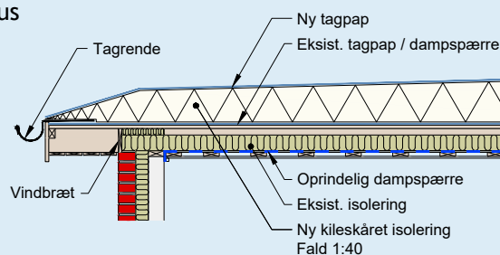
Fig. 2 Koldt tag: Udvendig merisolering af koldt tag med en ny udvendig tagrende, så høj sternkant undgås.
